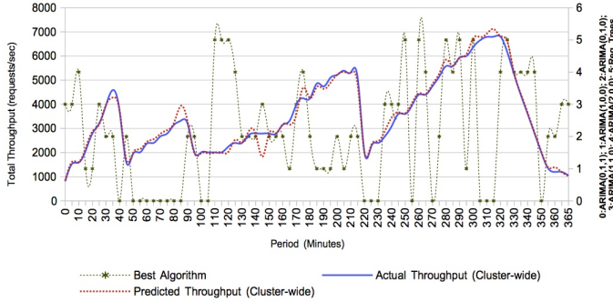
Fig. 10: Actual workload V.S. predicted workload
